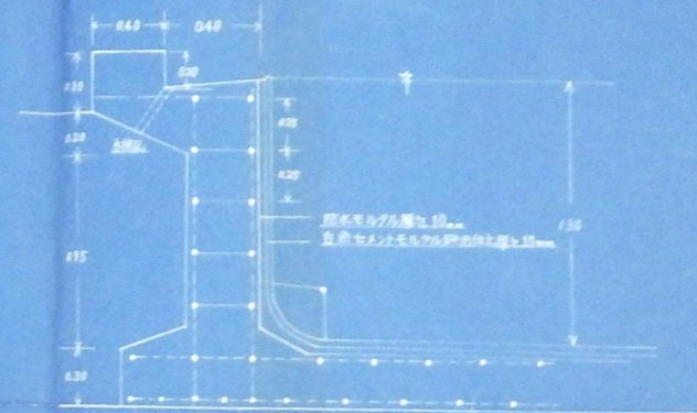
プール側壁断面図 1/20
